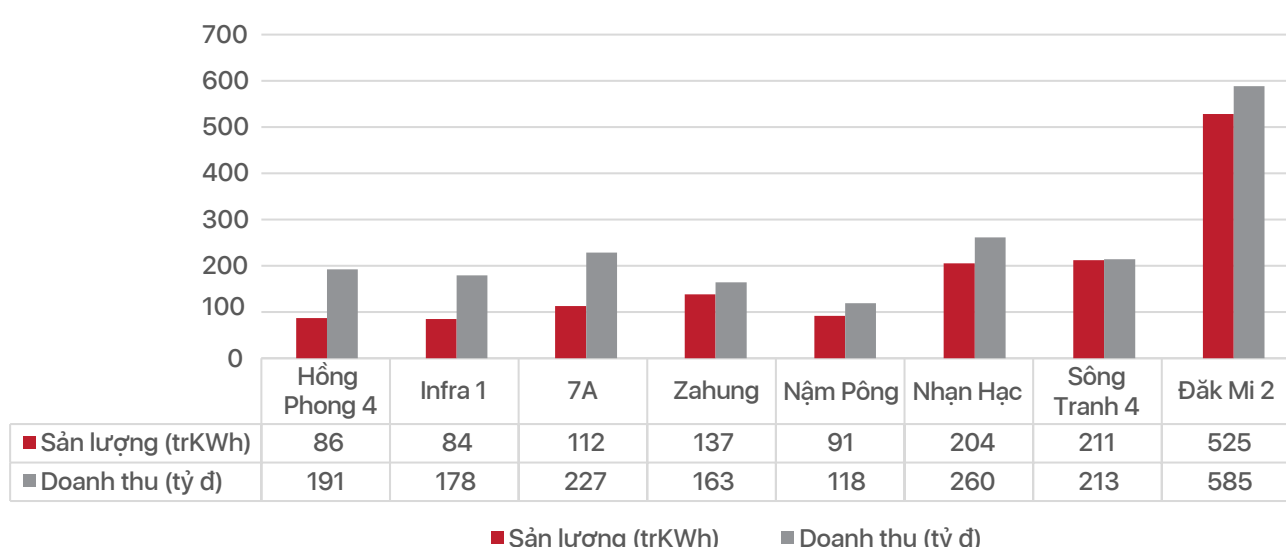
Sản lượng & doanh thu các nhà máy điện năm 2023
